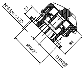
Sez. G-G
