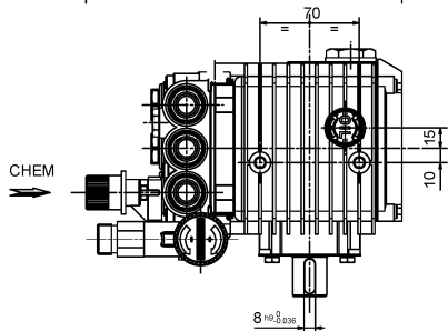
Sez. G-G
